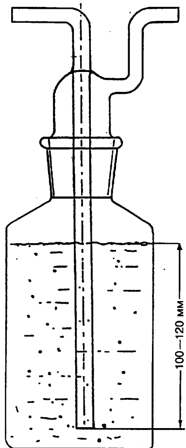
Рисунок 2 - Сосуд-смеситель
